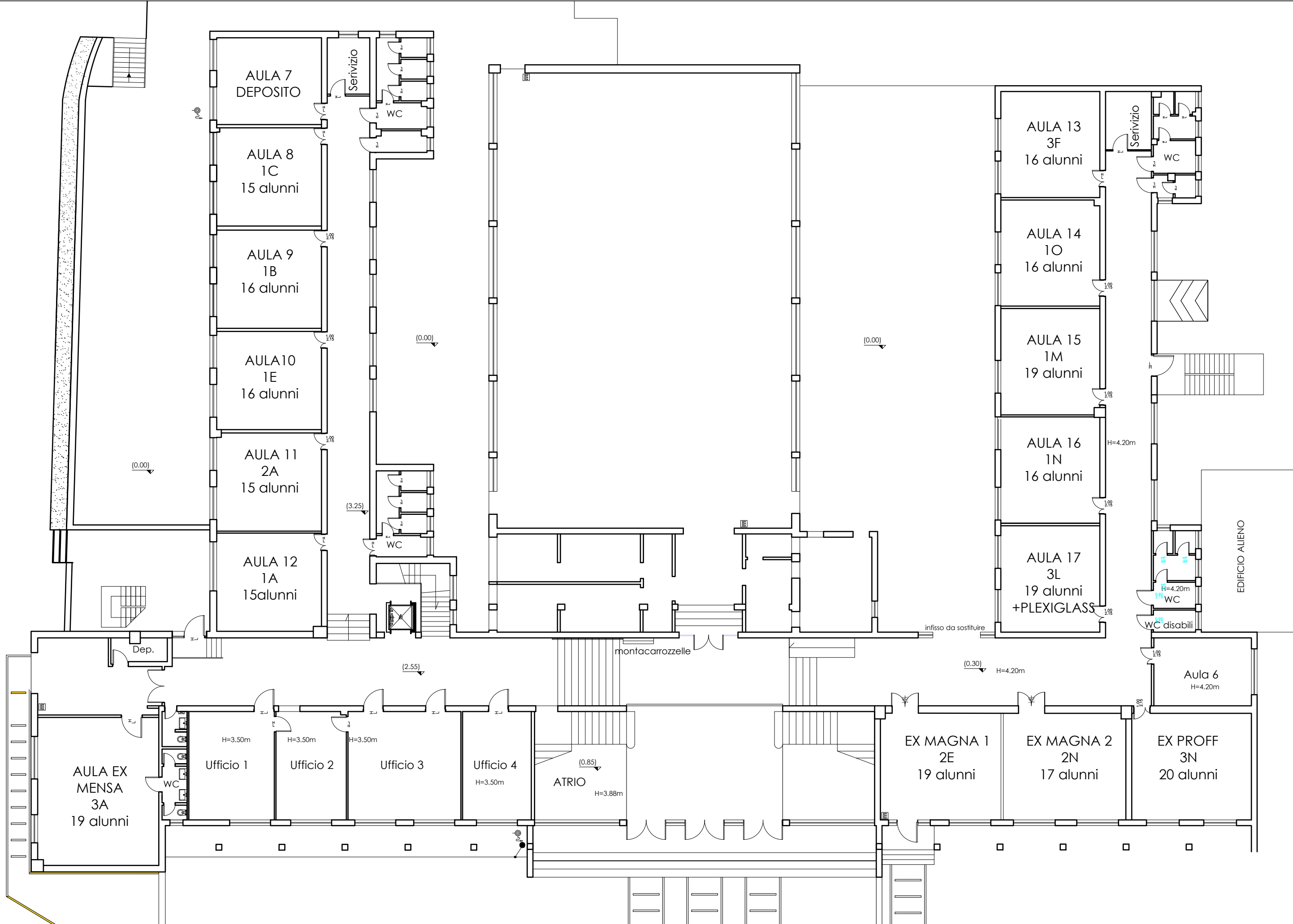
ISTITUTO SECONDARIO DI PRIMO GRADO "G. SCOTTI" ISCHIA- DISPOSIZIONE CLASSI: PIANO TERRA. - FUORI SCALA
